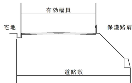
(3) 防護柵を設ける場合
